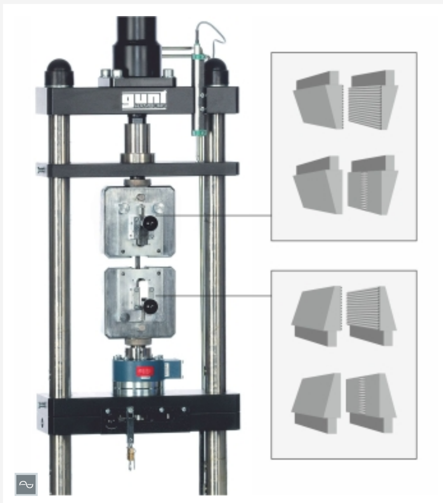
Die Abbildung zeigt beide Spannvorrichtungen mit Beißeilen für Rundproben und Beißeilen für Flachproben
