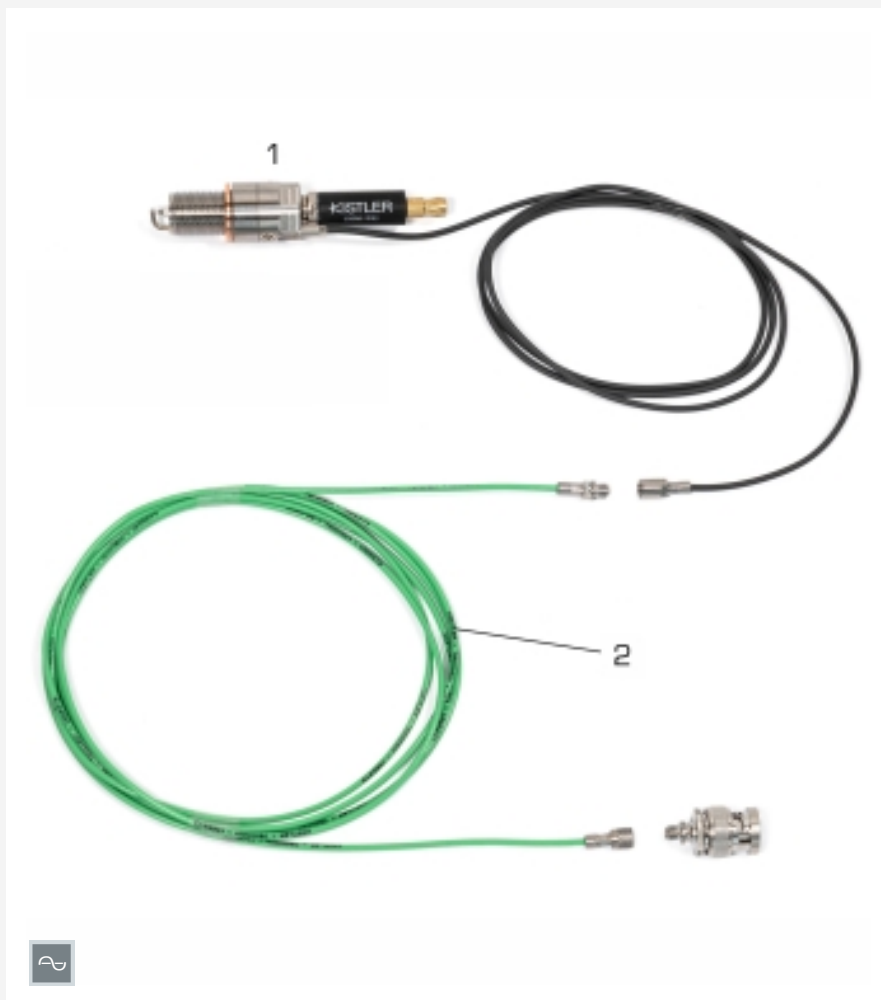
1 bougie avec capteur de pression, 2 câble de connexion
