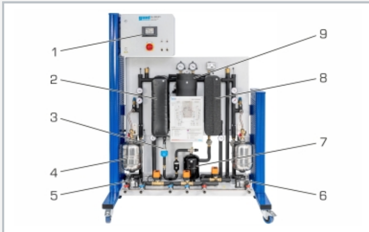
1 frei programmierbarer Heizungsregler: Bedienung über Touchscreen oder Webbrowser, 2 Verdampfer, 3 Expansionsventil, 4 Ausdehnungsgefäß, 5 Pumpe Quellkreislauf, 6 Pumpe Heizkreislauf, 7 Sammler, 8 Verflüssiger, 9 Scrollverdichter
