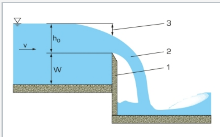
Nappe dénoyée au niveau du déversoir à paroi mince: 1 déversoir à paroi mince, 2 lame déversante, 3 abaissement; v vitesse d'écoulement, h_0 hauteur, W hauteur du déversoir
