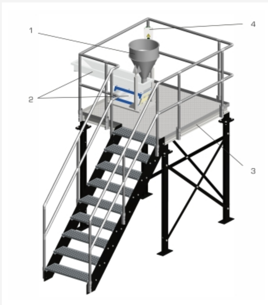
1 entonnoir, 2 alimentateur avec goulotte d'alimentation vibrante, 3 estrade, 4 boîte de raccordement
