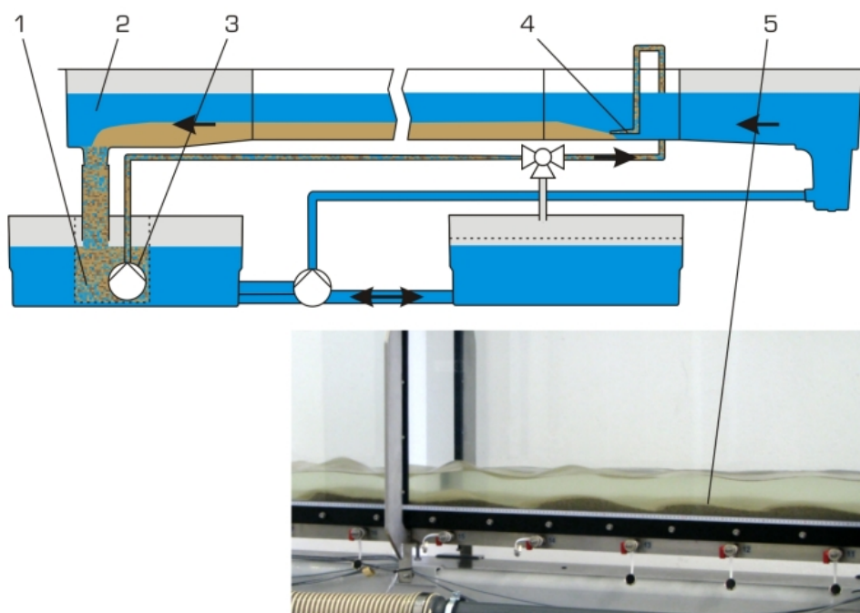
1 crépine, 2 élément de sortie du HM 163, 3 pompe, 4 alimentateur en sédiments, 5 déplacement des dunes
