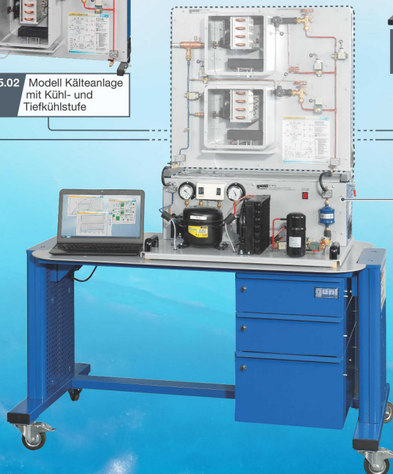
die Basiseinheit ET 915 enthält die Hauptkomponenten Verdichter und Verflüssiger
