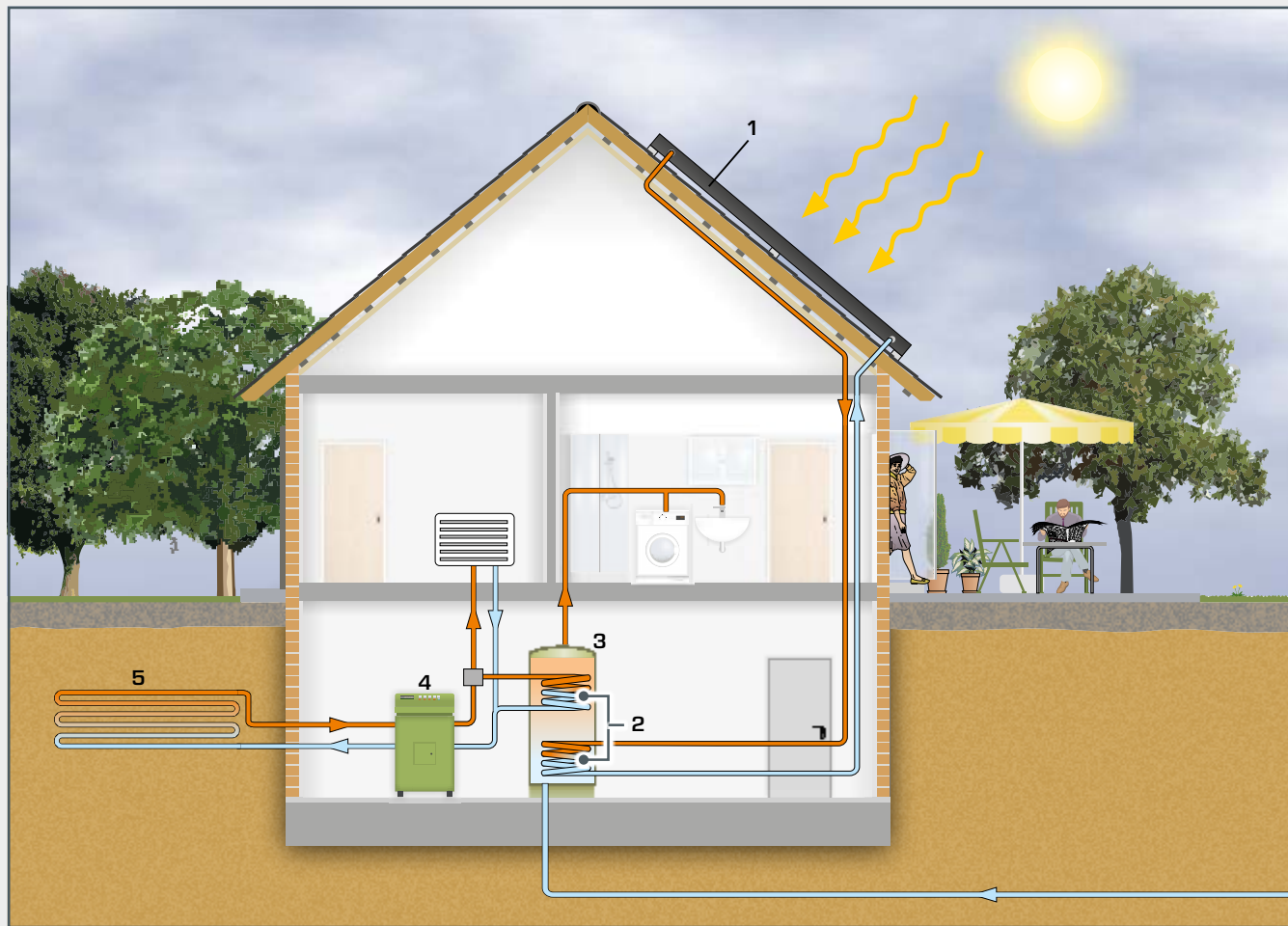
1 Flachkollektor, 2 Wärmeübertrager, 3 Warmwasserspeicher, 4 Wärmepumpe, 5 Erdwärmeabsorber; orange warme Wärmeträgerflüssigkeit, blue kalte Wärmeträgerflüssigkeit, red Kältemittel Hochdruckseite, blue Kältemittel Niederdruckseite
