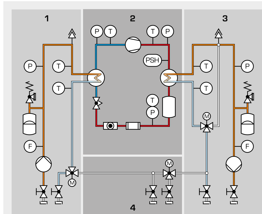
Prozessschema des Moduls HL 320.01 Wärmepumpe
