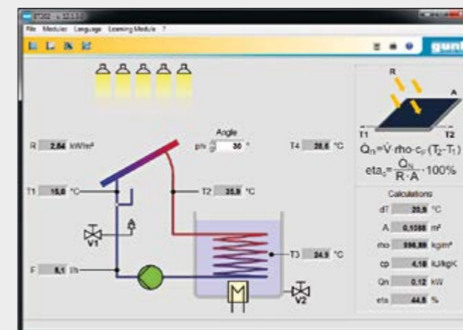
Logiciel GUNT pour l'acquisition des données de mesure via un PC
