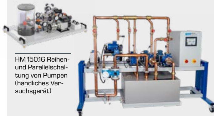
HM 362 Vergleich von Pumpen (komplexer Versuchstand)
